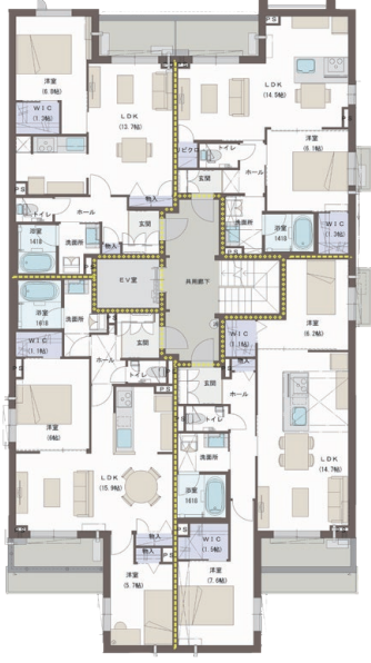
2・3階平面図
